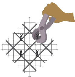
A tela é amarrada na malha com arame recozido, utilizando a Turquesa a cada dois quadros
